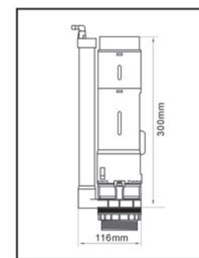
MOULD:A-2006
