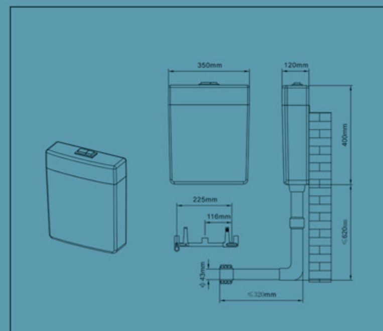
MOULD:A-7100
