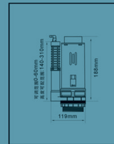
MOULD:A-2112
